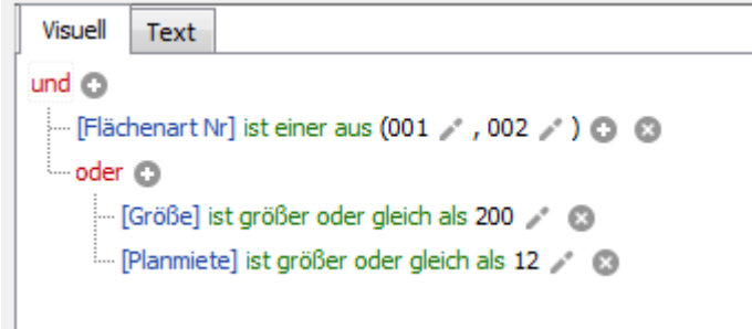
Abb. 2: Beispiel für Definition von Kriterien für Alarmregeln
