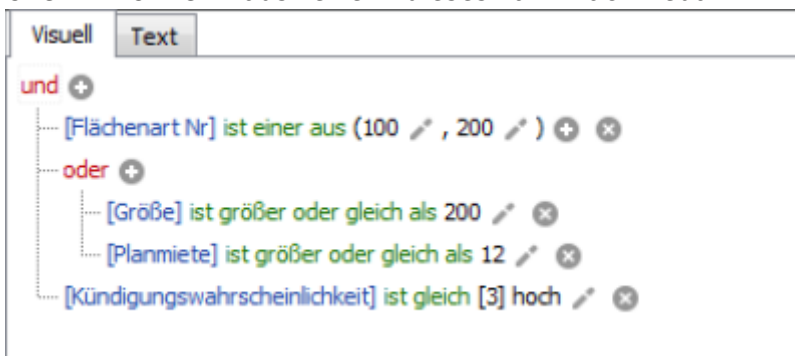
Abb.: Beispiel für Alarmregeln unter Berücksichtigung einer Kündigungswahrscheinlichkeit
